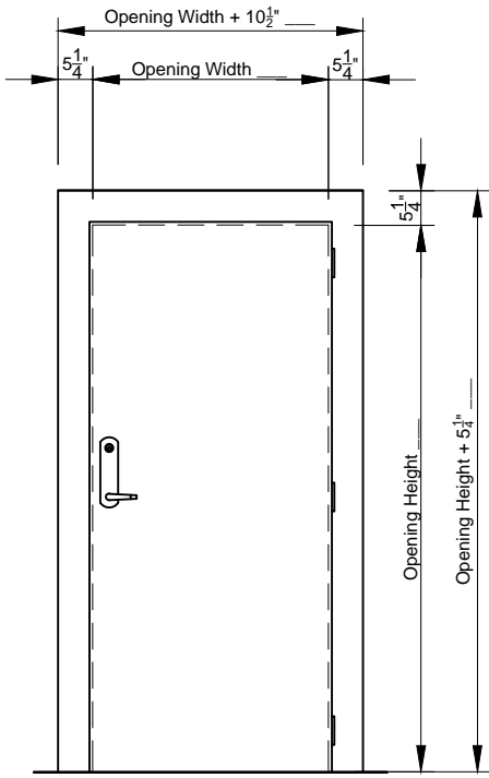
① SCALE: 3/8" = 1'-0"
